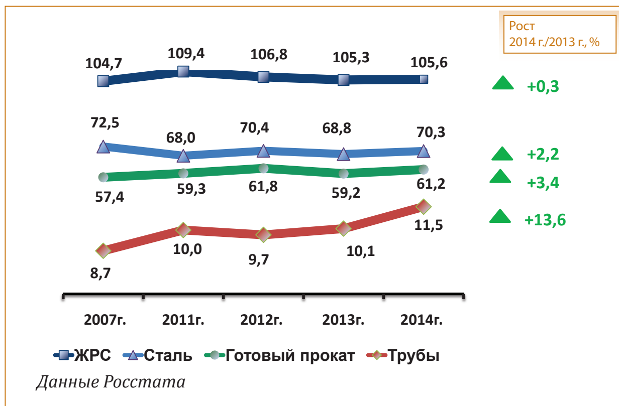
Динамика объемов производства основных видов продукции черной металлургии (Млн. тонн)
